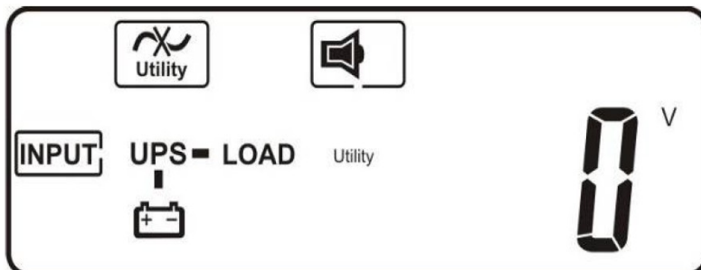
Рис. I ИБП включен «Холодным стартом». Входное напряжение отсутствует.
