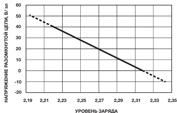
Рис. 6. Рекомендуемое напряжение поддерживающего заряда AGM батарей при различных уровнях температуры окружающей среды
