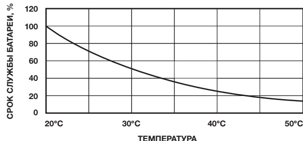
Рис. 4. Ожидаемый срок службы в зависимости от температуры
