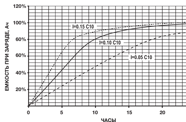
Рис.7. Кривые заряда AGM батарей FIAMM при напряжении 2,4 В/эл. с различными пределами зарядного тока.
