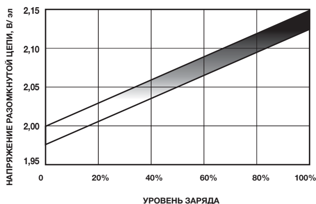
Рис.5 Приблизительный уровень заряда в зависимости от напряжения разомкнутой цепи AGM аккумулятора FIAMM
