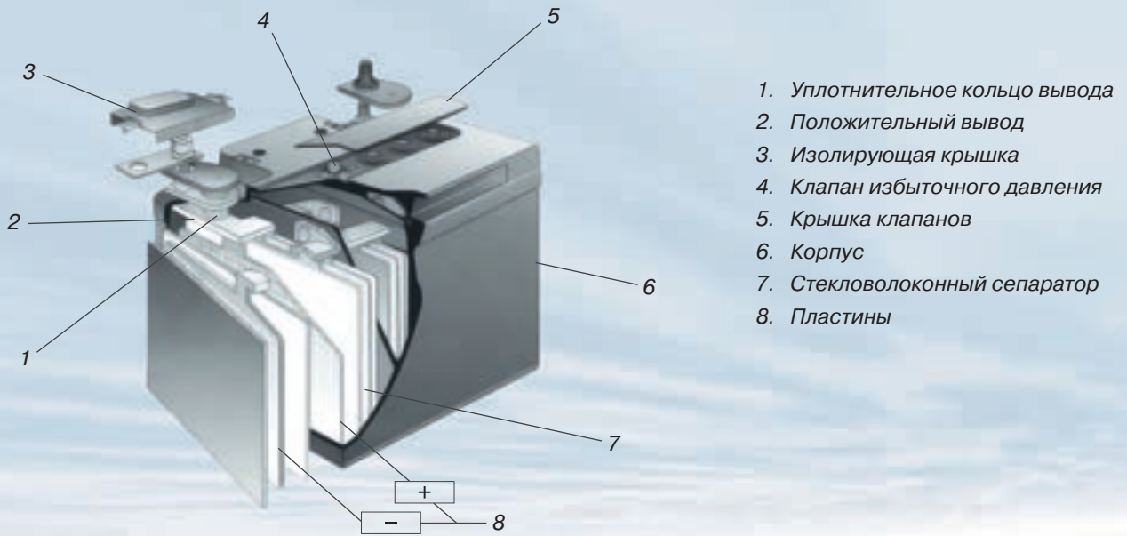
Рис. 1 Общее устройство аккумуляторов
