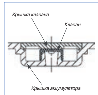
Рис. 3 Клапан избыточного давления
