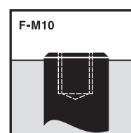
Винт FM10, 17 Nm
