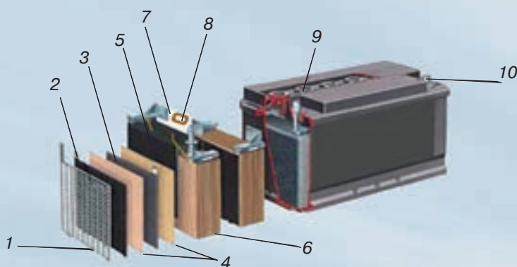
Рис. 1 Общее устройство аккумулятора
