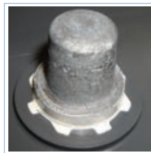
Рис. 4 Конусный вывод
