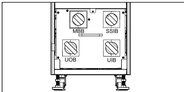
ИБП мощностью 60-100 кВА с внешними батареями
