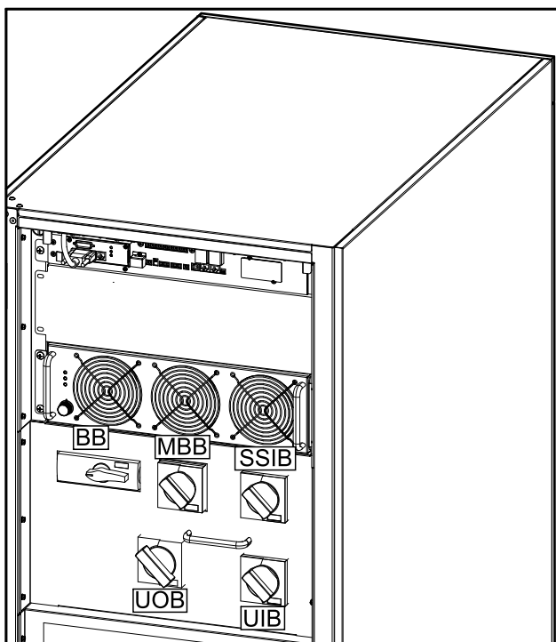
ИБП мощностью 60 кВА с внутренними батареями, вид спереди
