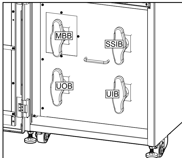
ИБП мощностью 200 кВА с внешними батареями
