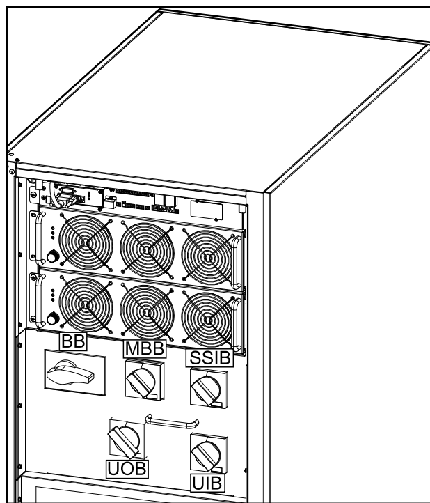
ИБП мощностью 80 кВА с внешними батареями, вид спереди
