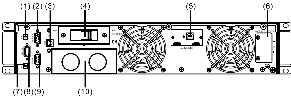
Задняя панель ИБП Monolith V 6-10кВА
