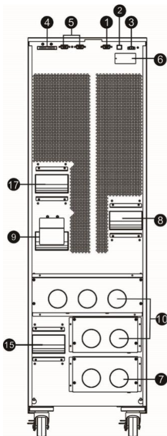
Рисунок 9 Вид сзади PM60
