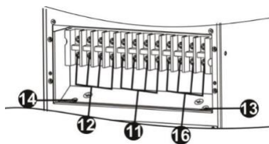
Рисунок 4 Клеммная колодка вход/выход с отдельным входом байпаса ONTEK PM10/10SB/15/15SB/20/20SB
