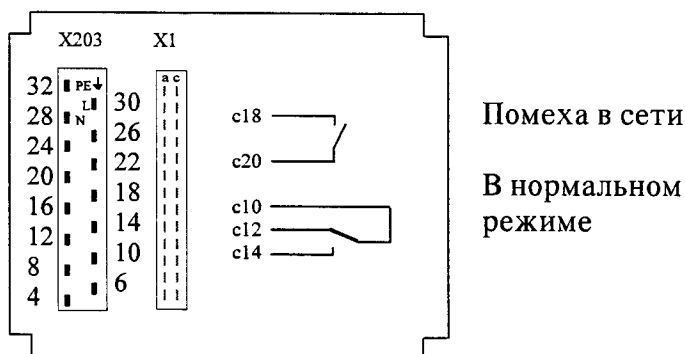
Рисунок 12. Подключение выпрямителя.
