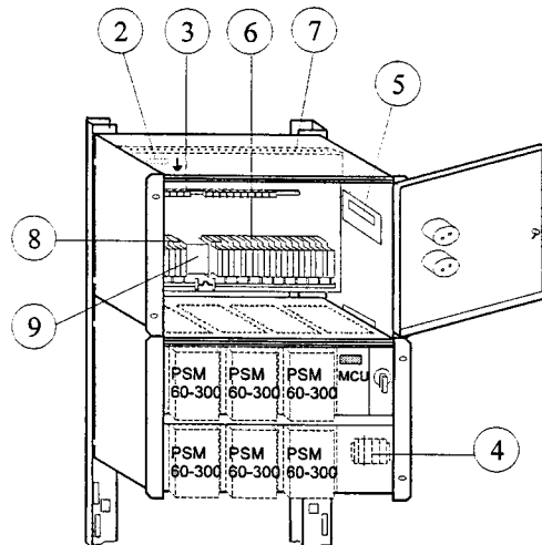
Рисунок 5. Модульный каркас SCM 60-300.6
