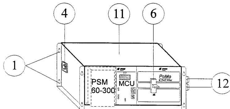
Рисунок 2. Каркасный модуль 60-300.1
