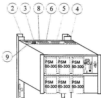
Рисунок 7. Модульный каркас SCM 60-300.6V
