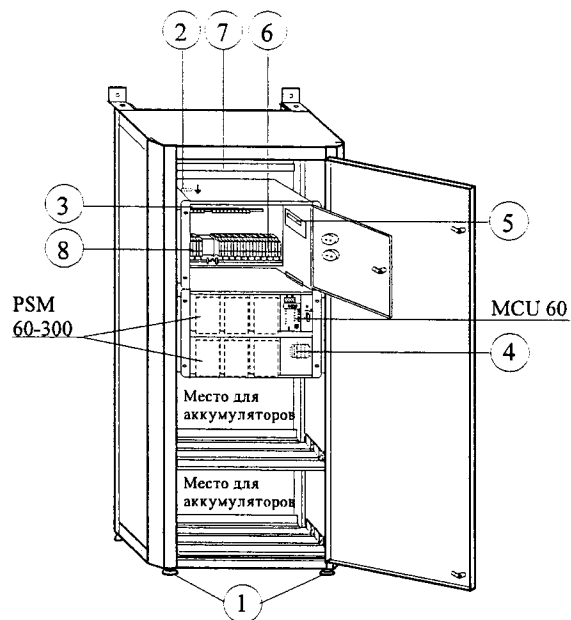
Рисунок 10. Модульный каркас SCM 60-300.6C1
