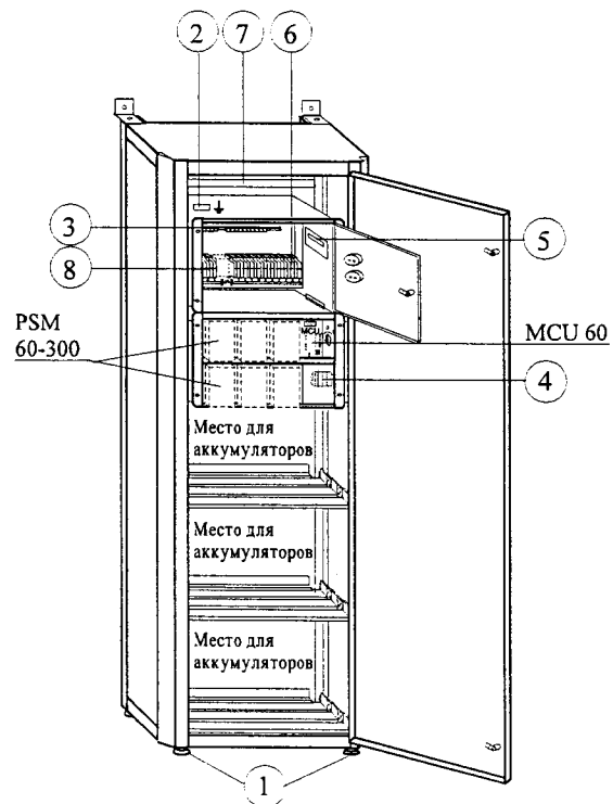
Рисунок 11. Модульный каркас SCM 60-300.6C2
