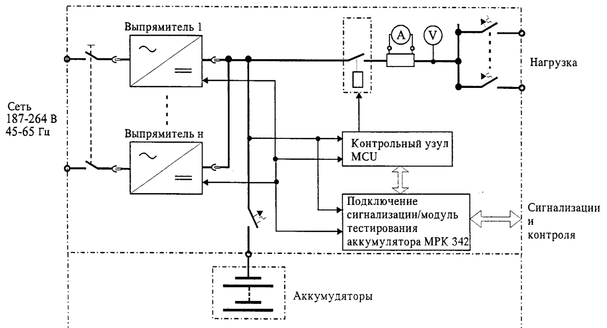
Рисунок 1. Системы PoMo 60-300.xx
