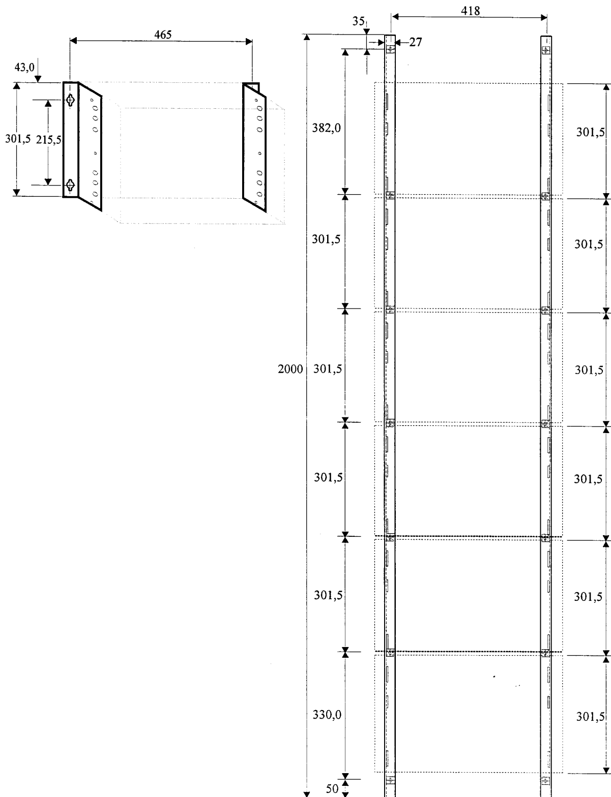
Рисунок 3. Настенные рельсы и уголки.
