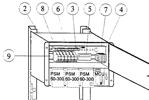
Рисунок 6. Модульный каркас SCM 60-300.3
